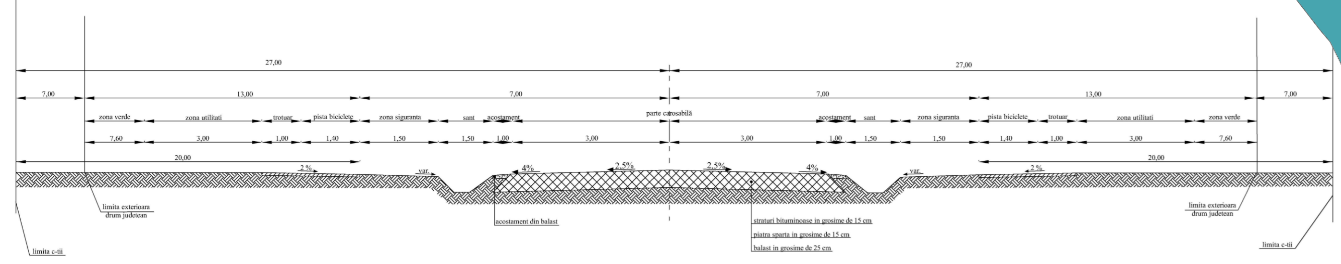
PROFIL TRANSVERSAL DJ 503 KM 51+417m la KM 52+434m KM 53+596m la KM 54+026m
